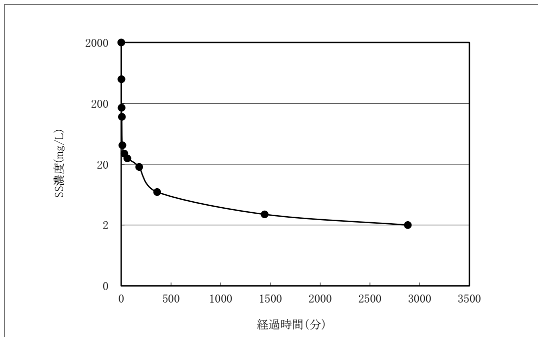
图 10.4-2(2) 土壤沉降試驗結果 (地点⑧)
